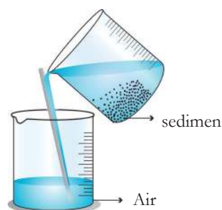
Gambar 5.25 Metode dekantasi.
