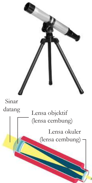
Gambar 4.11 Teknologi Teleskop
