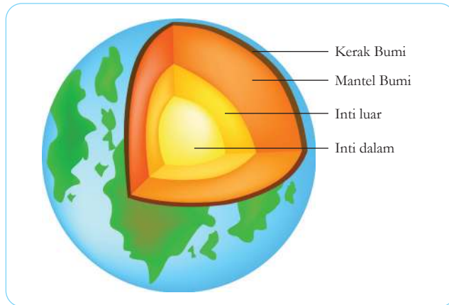
Gambar 6.3 Struktur bumi
